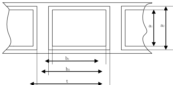
图 1 画幅 ( a_2 \times b_2 )、影像区 ( a_1 \times b_1 ) 和进片距 ( t )
